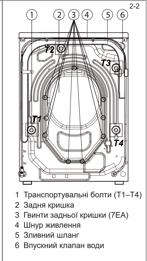
Вигляд ззаду (рис. 2-2)
