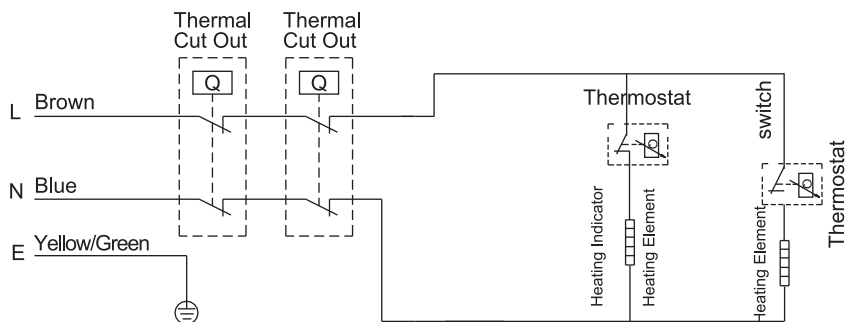
СХЕМА ЕЛЕКТРОПРОВІДКИ
