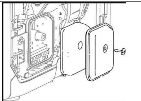
Зняття кришки повітряного фільтра
