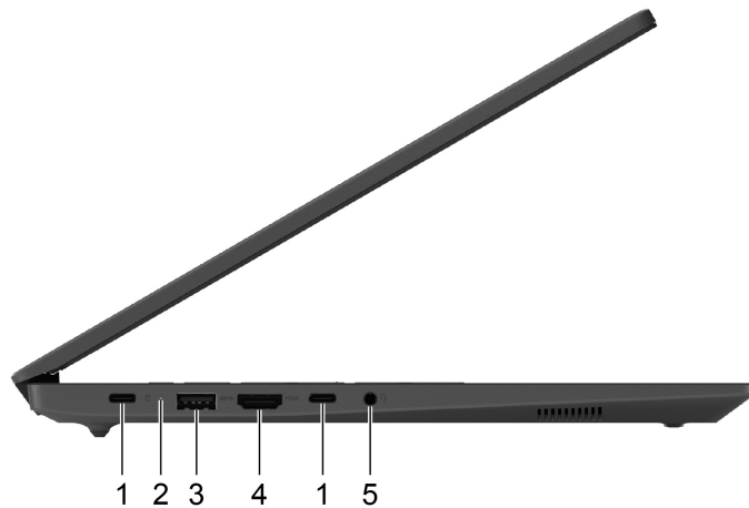
Малюнок 5. Моделі 15 дюймів—вид зліва
