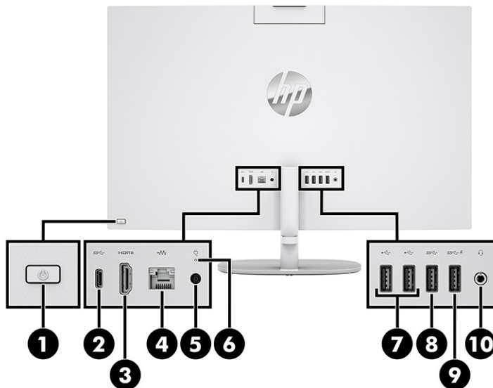
Таблиця 4-2 Визначення компонентів задньої панелі
