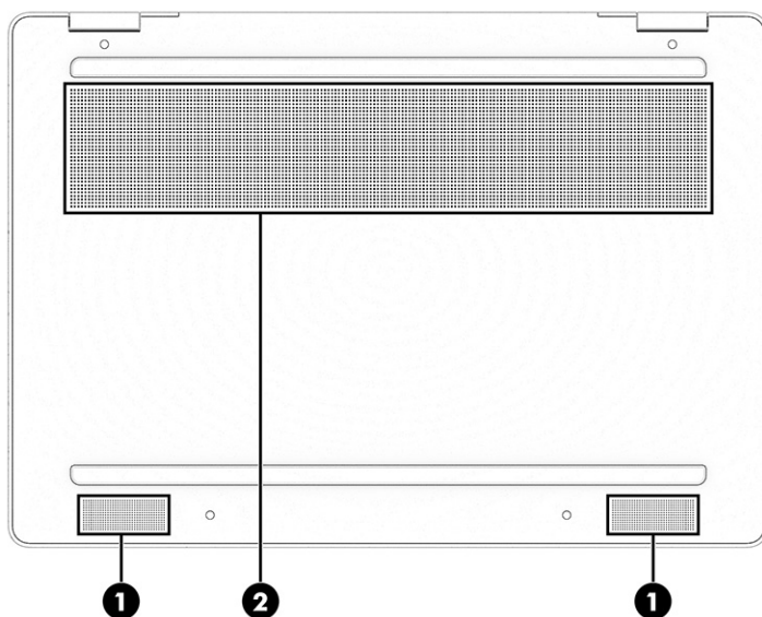
Таблиця 3-8 Компоненти нижньої панелі та їх опис
