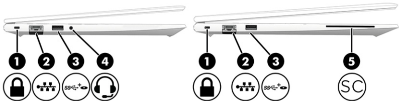
Таблиця 2-2 Компоненти лівої панелі та їх опис
