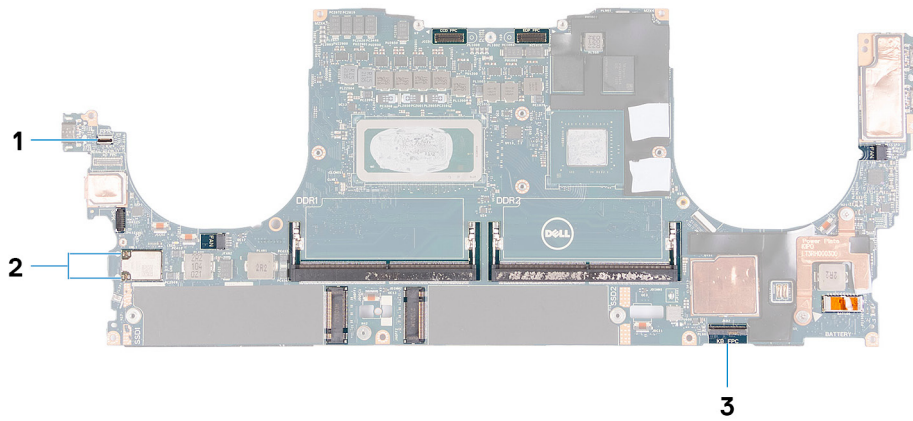
Рисунок 2. Разъемы на системной плате
