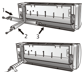
Згортання з'єднувального патрубка
